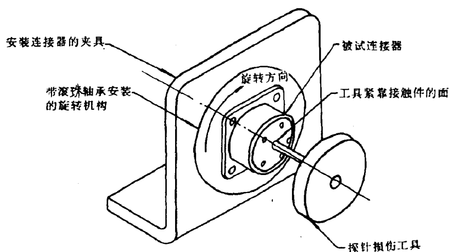
装置 2 在连接器里试验插孔接触件用的设备
