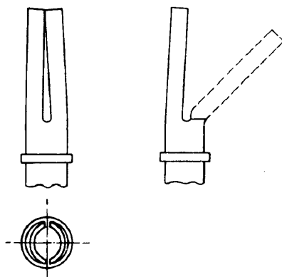
图 6 双或多叉指插孔接触件
