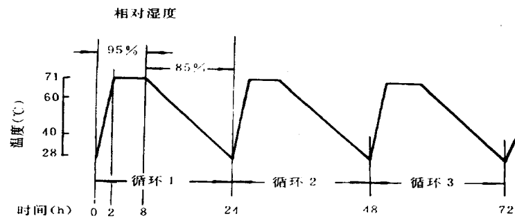
图 1 I 型交变湿热试验
