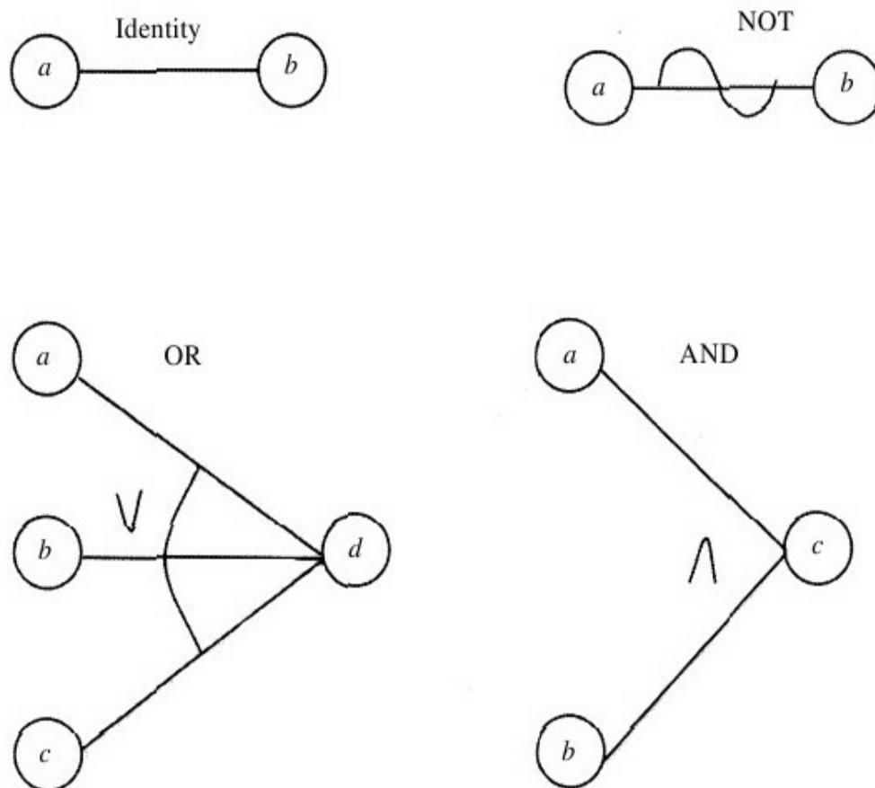
图 4-5 基本的因果图符号
