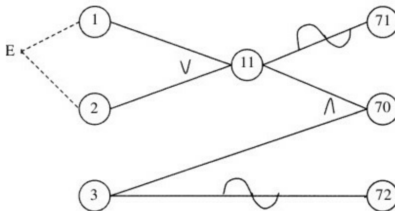
图 4-10 带有“排斥性”约束条件的因果图范例
