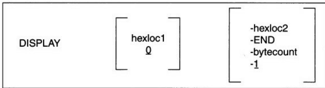
图 4-11 DISPLAY 命令的语法
