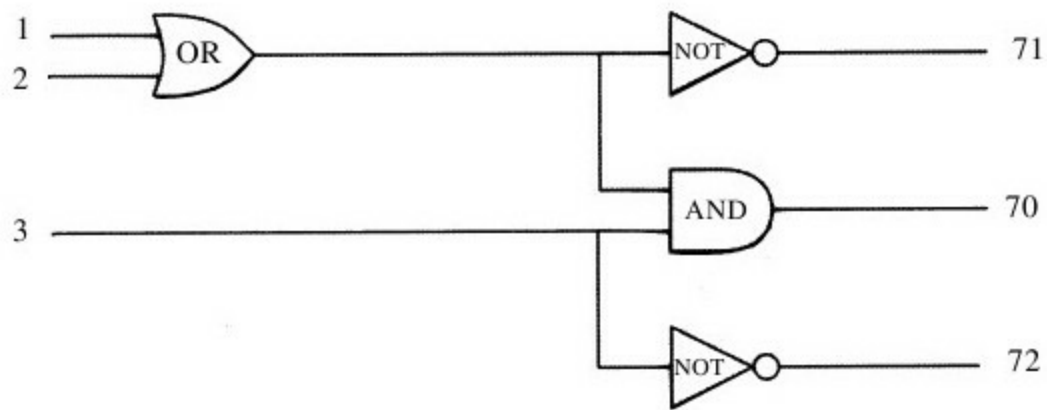
图 4-7 与图4-6等价的逻辑图
