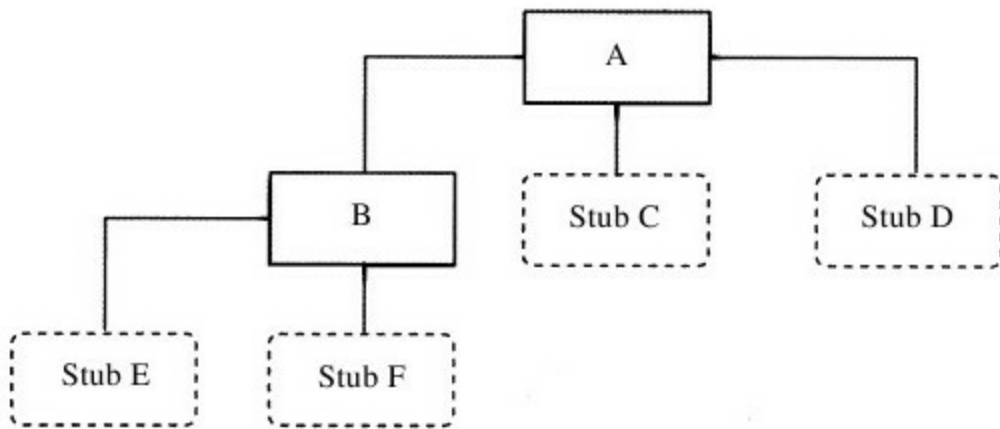
图 5-9 自顶向下测试的第二个步骤
