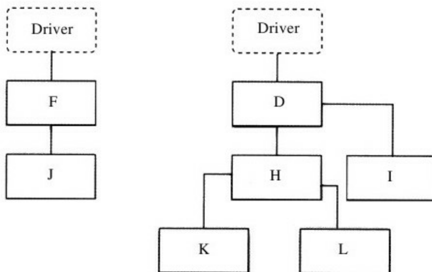
图 5-11 自底向上测试的中间状态
