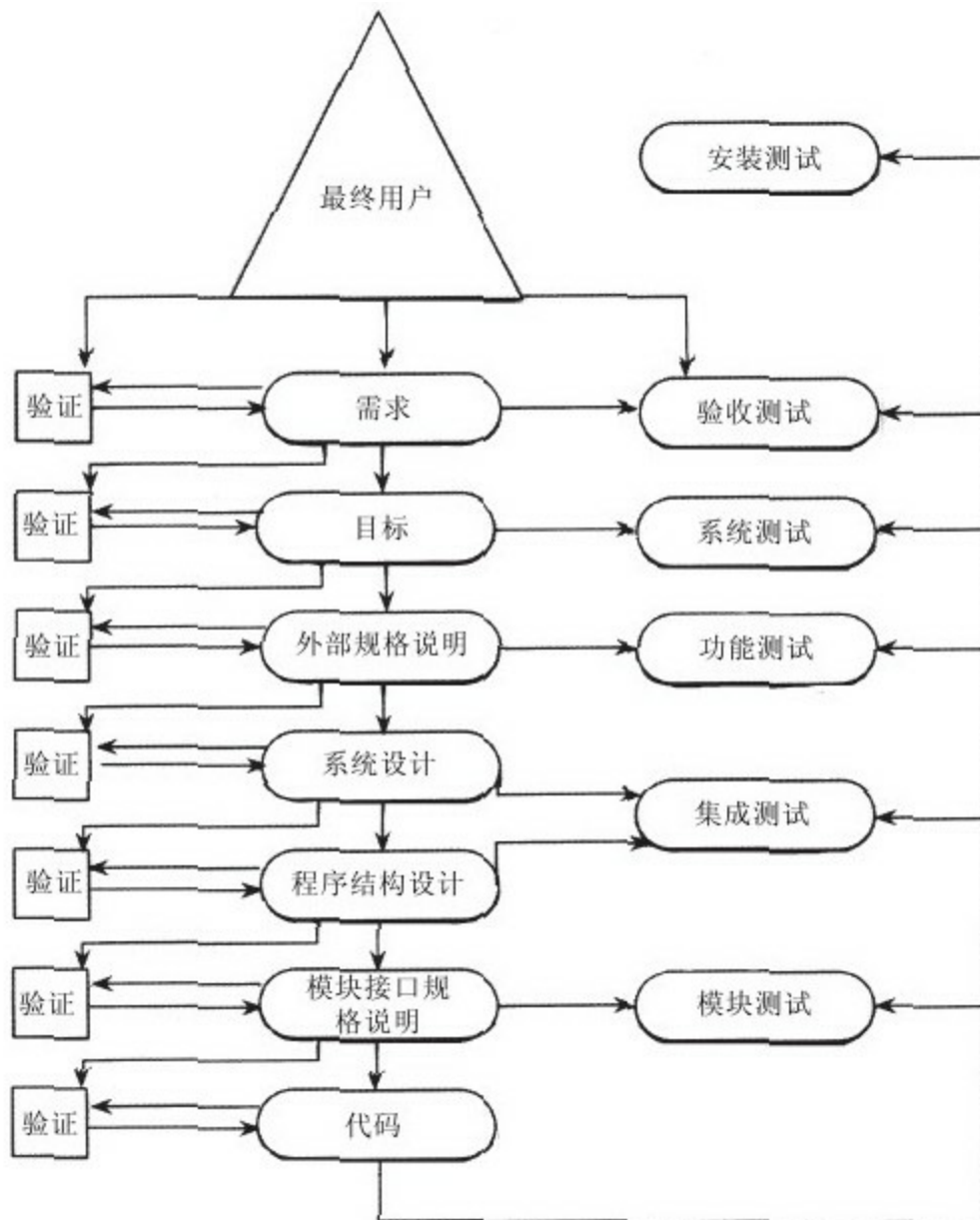
图 6-3 开发过程与测试过程的对应关系
