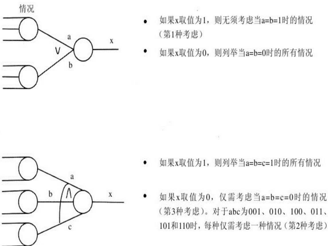
图 4-15 追溯因果图的思路
