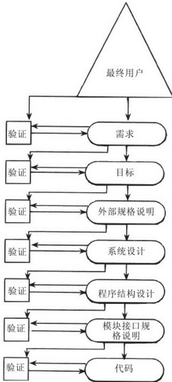
图 6-2 包含中间验证步骤的开发过程
