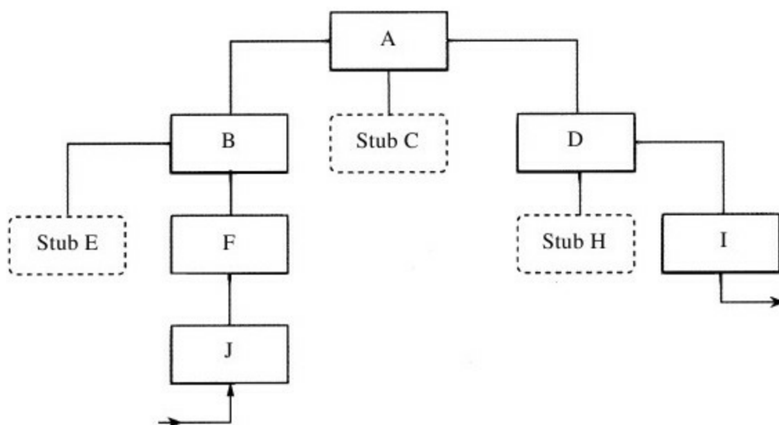
图 5-10 自顶向下测试的中间状态
