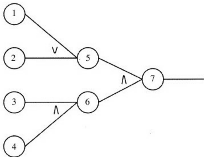
图 4-16 描述追溯思路的因果图范例
