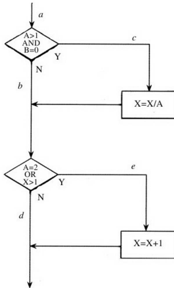
图 4-1 被测试的小程序
