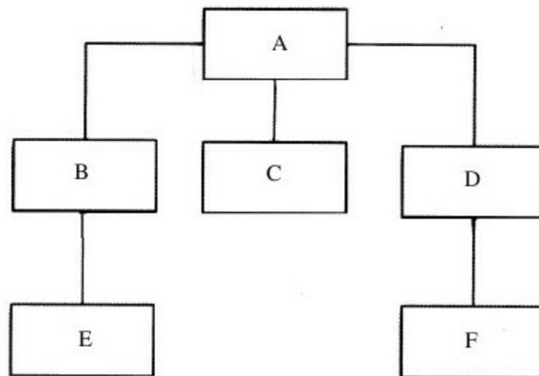
图 5-7 包含6个模块的程序范例
