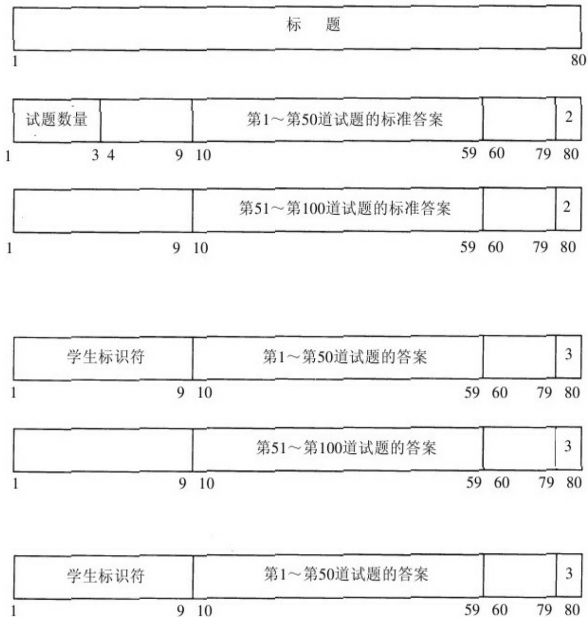
图 4-4 MTEST程序的输入
